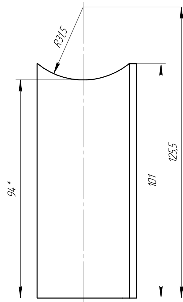
Дет. поз. 2
