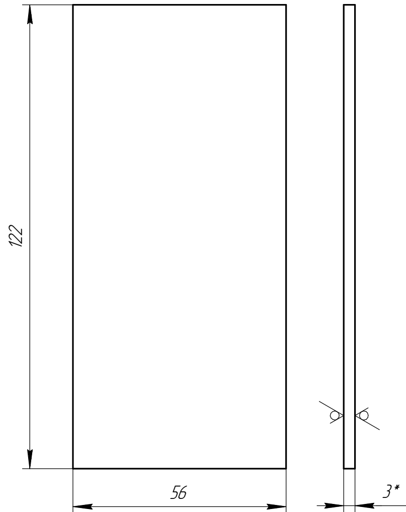
Дет. поз. 1
