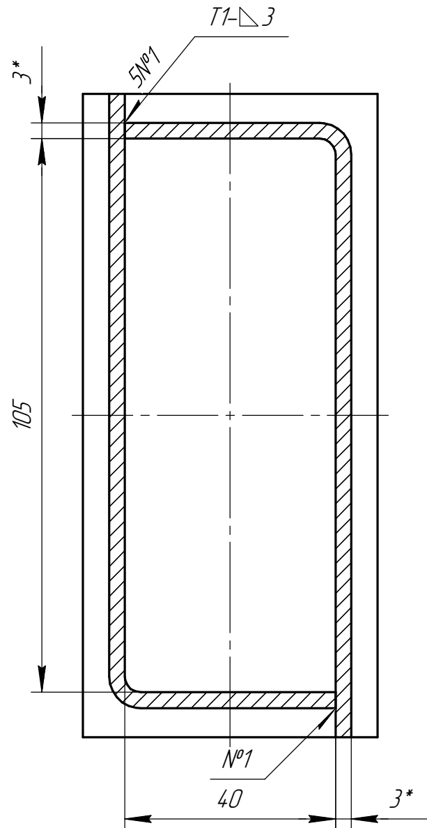
Б-Б
