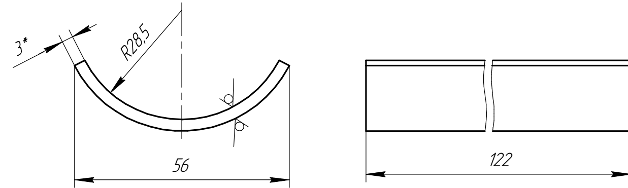
Дет. поз. 3
